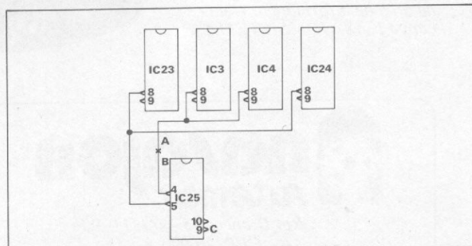
Figura 2 - Esquema da alteração
